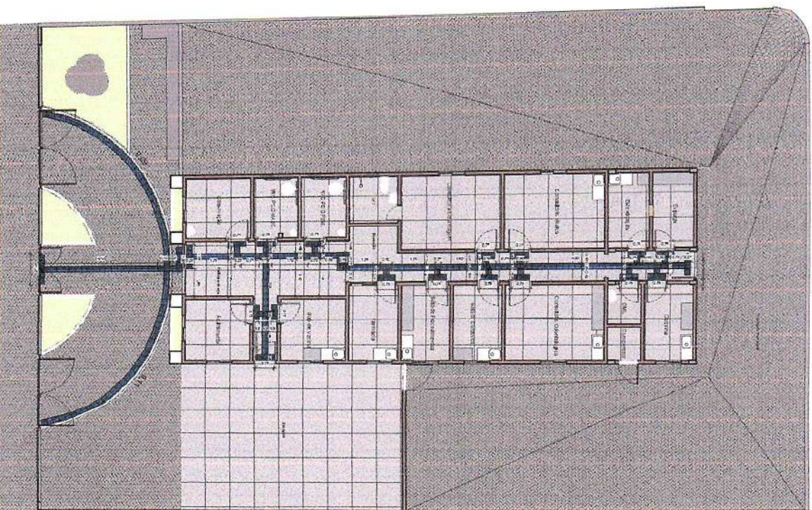
2 PLANTA - TÉRREO PISO TÁTIL Escala 1 : 75
